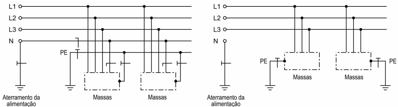
Figura 4 — Esquema TT
